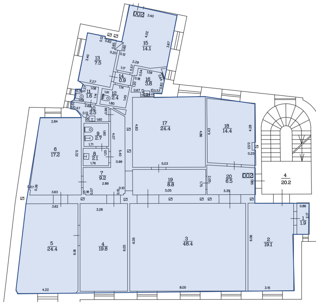
Telpu grupa 002, telpas Nr.1-20, ar kopējo platību 231,7 m²
